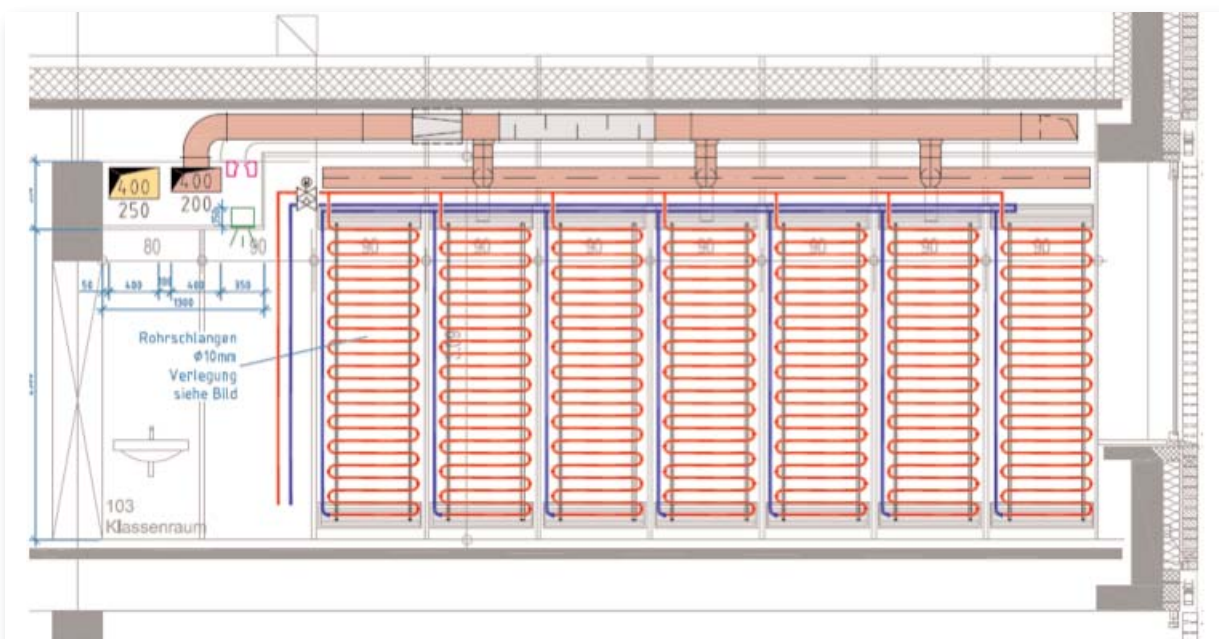
Abb. 8-5: Detailzeichnung der Klimawand
