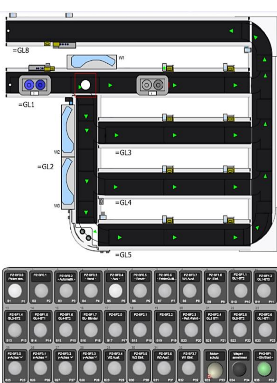
Anlagensimulation der Station Fertigung
