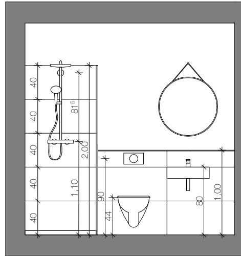
Ansicht A
