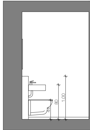
Ansicht B
