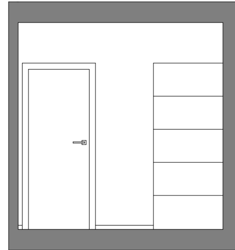
Ansicht C
