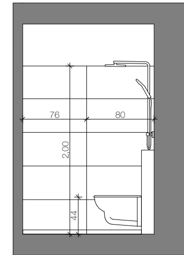
Ansicht D
