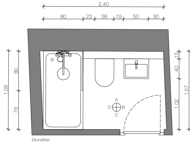
Grundriss
