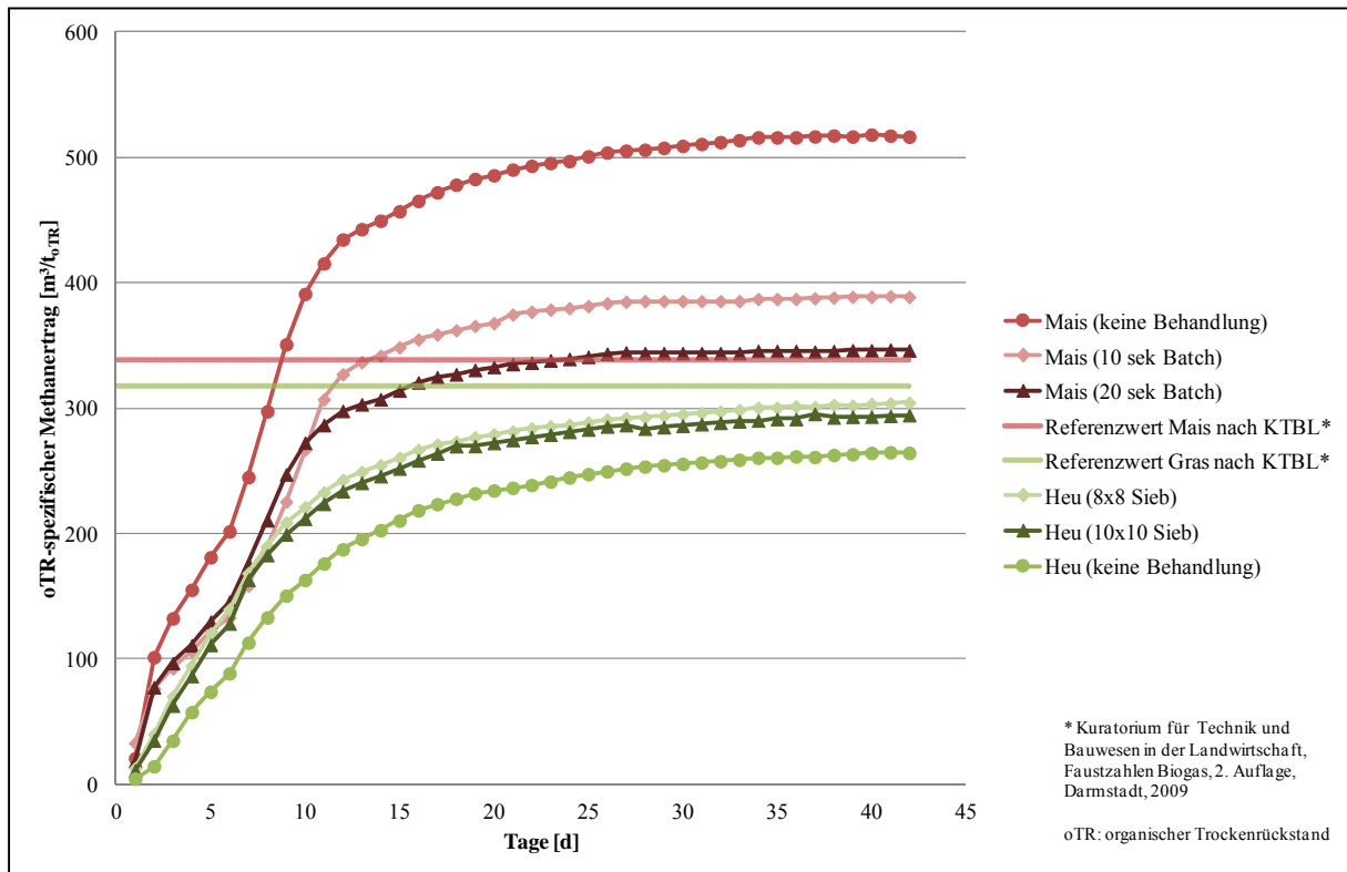
Abb. 4-14: oTR-spezifischer Methanertrag der Heu- und Maissilageproben
