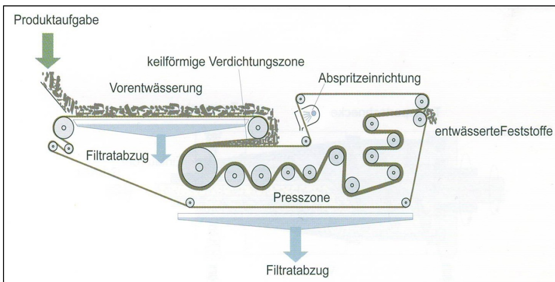
Abb. 10-2: Schematische Darstellung einer Bandfilterpresse [20]
