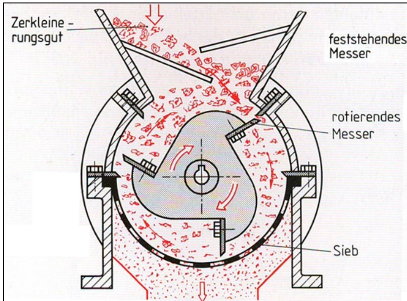
Abb. 4-1: Schematische Darstellung einer Schneidmühle [7]
