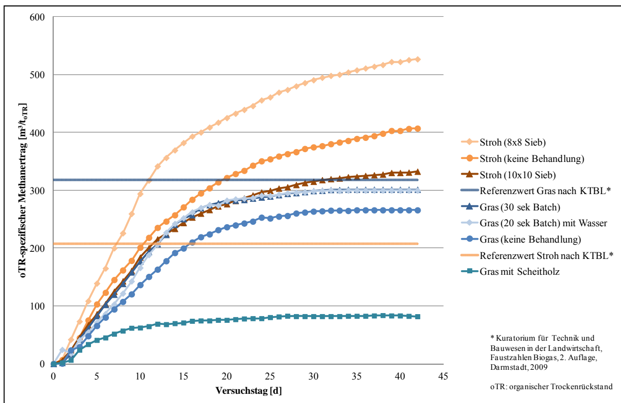
Abb. 4-13: oTR-spezifischer Methanertrag der Stroh- und Grassilageproben
