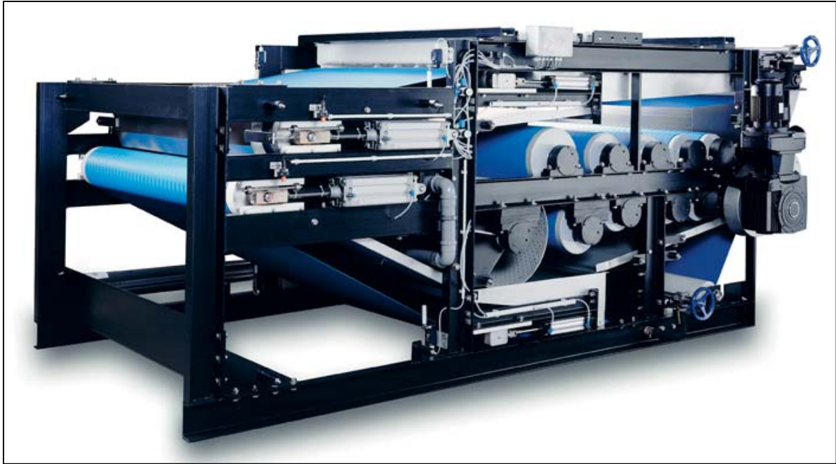
Abb. 10-1: Bandfilterpresse der Fa. Klein [19]
