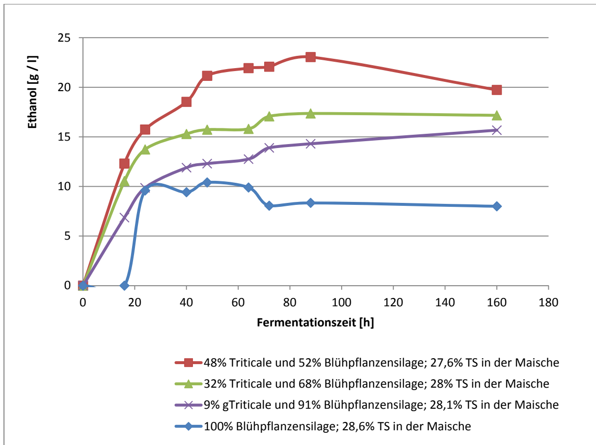
Abb. 6-8: Vergärung einer Blühpflanzensilagemaische, 6 Tage hydrolysiert, mit Triticalemaischevorhydrolysat vermengt. Die Prozentzahlen der einzelnen Kurvennamen geben das prozentuale Gewichtsverhältnis zwischen Lignocellulose- und Stärkefrucht an
