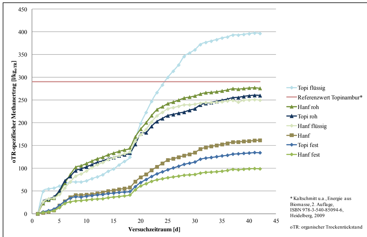
Abb. 8-5: oTR-spezifischer Methanertrag der Hanf-Triticale- und Topinambur-Triticale-Fractionen nach Schwingsieb mit 1,52 mm Maschenweite
