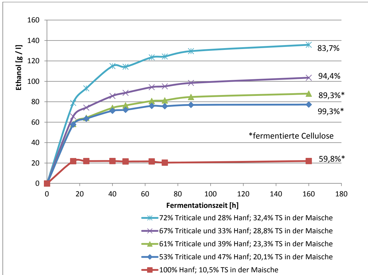
Abb. 6-7: Vergärung von Hanfstrohmaische 3,5 Tage hydrolysiert mit Triticalemaishevorhydrolysat vermengt. Die Prozentzahlen der einzelnen Kurvennamen geben das prozentuale Gewichtsverhältnis zwischen Lignocellulose- und Stärkefrucht an
