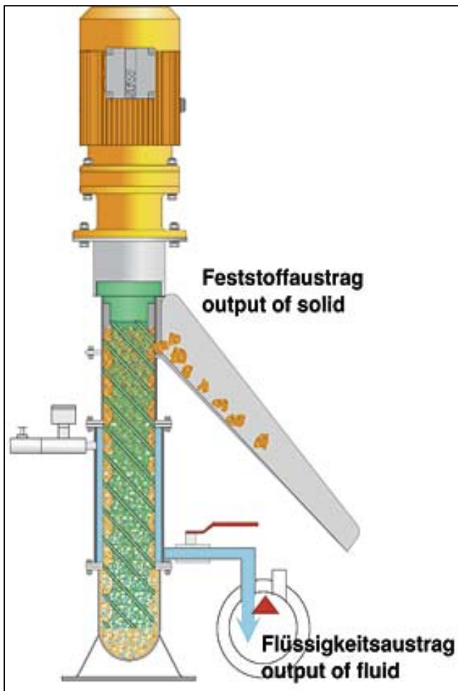
Abb. 10-8: Schemazeichnung des Klass-Wendelfilters [23]
