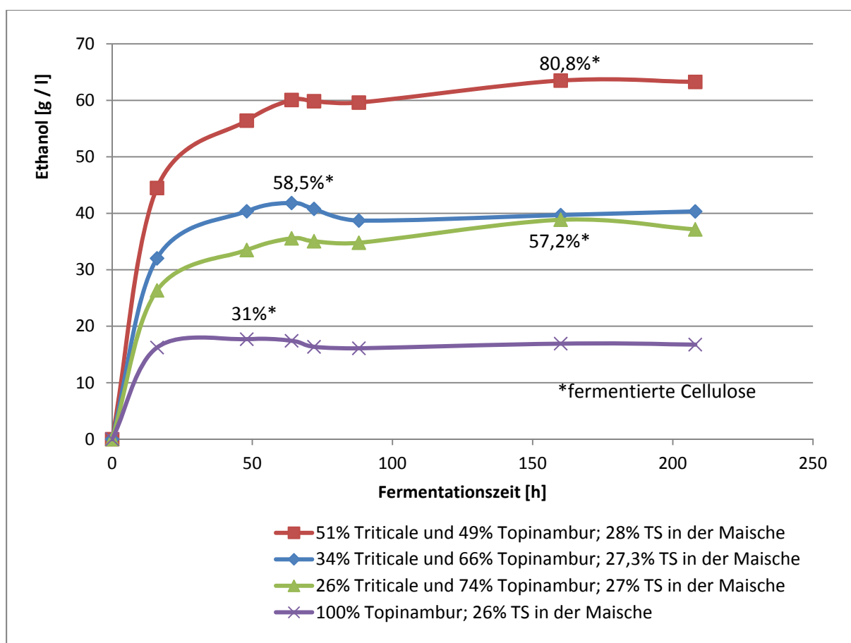
Abb. 6-3: Vergärung von Topinamburmaisichen 3 Tage hydrolysiert mit Triticalemaisichevorhydrolysat vermengt. Die Prozentzahlen der einzelnen Kurvennamen geben das prozentuale Gewichtsverhältnis zwischen Lignocellulose- und Stärkefrucht an
