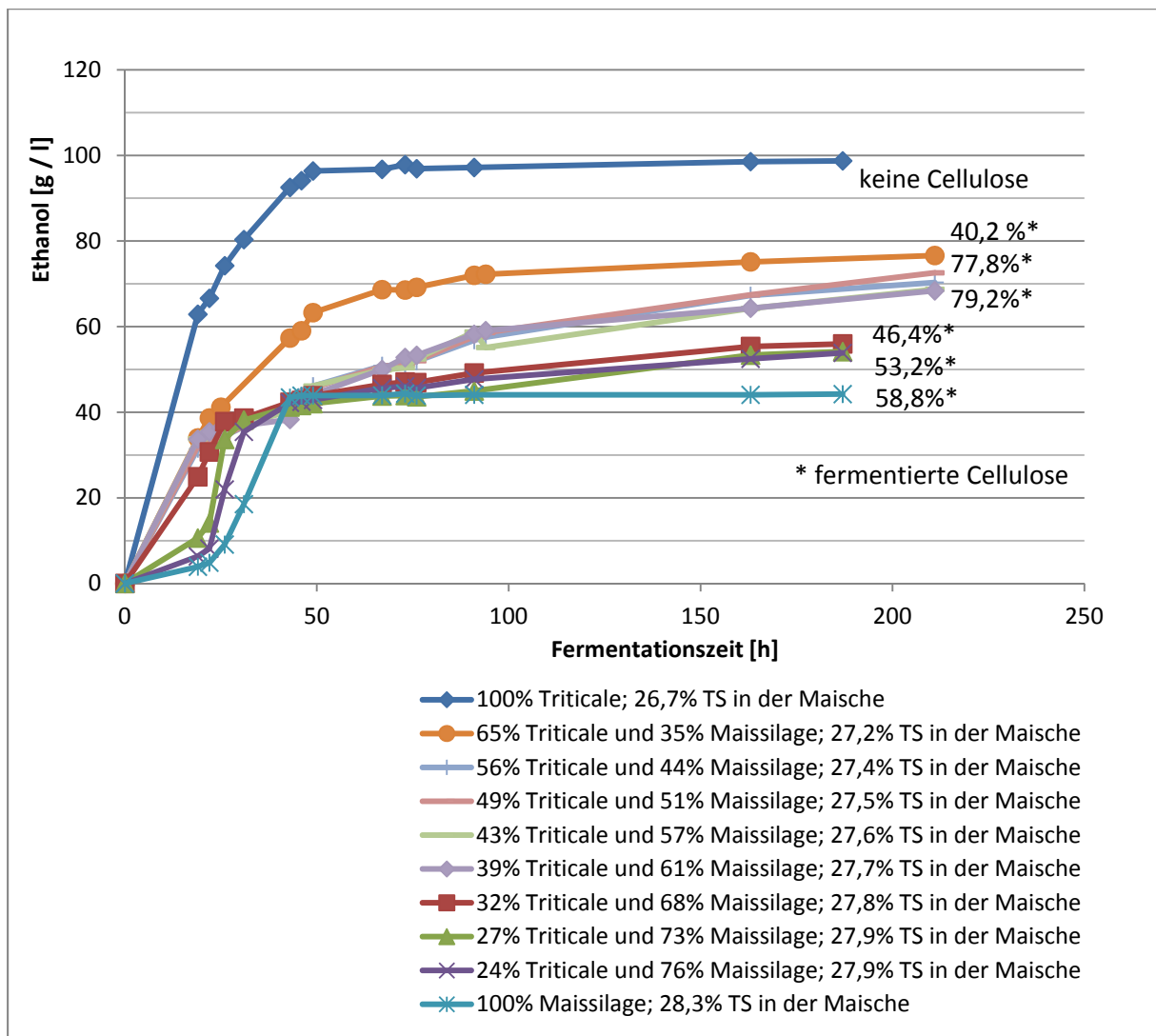
Abb. 6-1: Vergärung von Maissilagehydrolysat (28,6 % TS) mit Triticalemaischedydrolysat vermischt. Die Prozentzahlen der einzelnen Kurvennamen geben das prozentuale Gewichtsverhältnis zwischen Lignocellulose- und Stärkefrucht an
