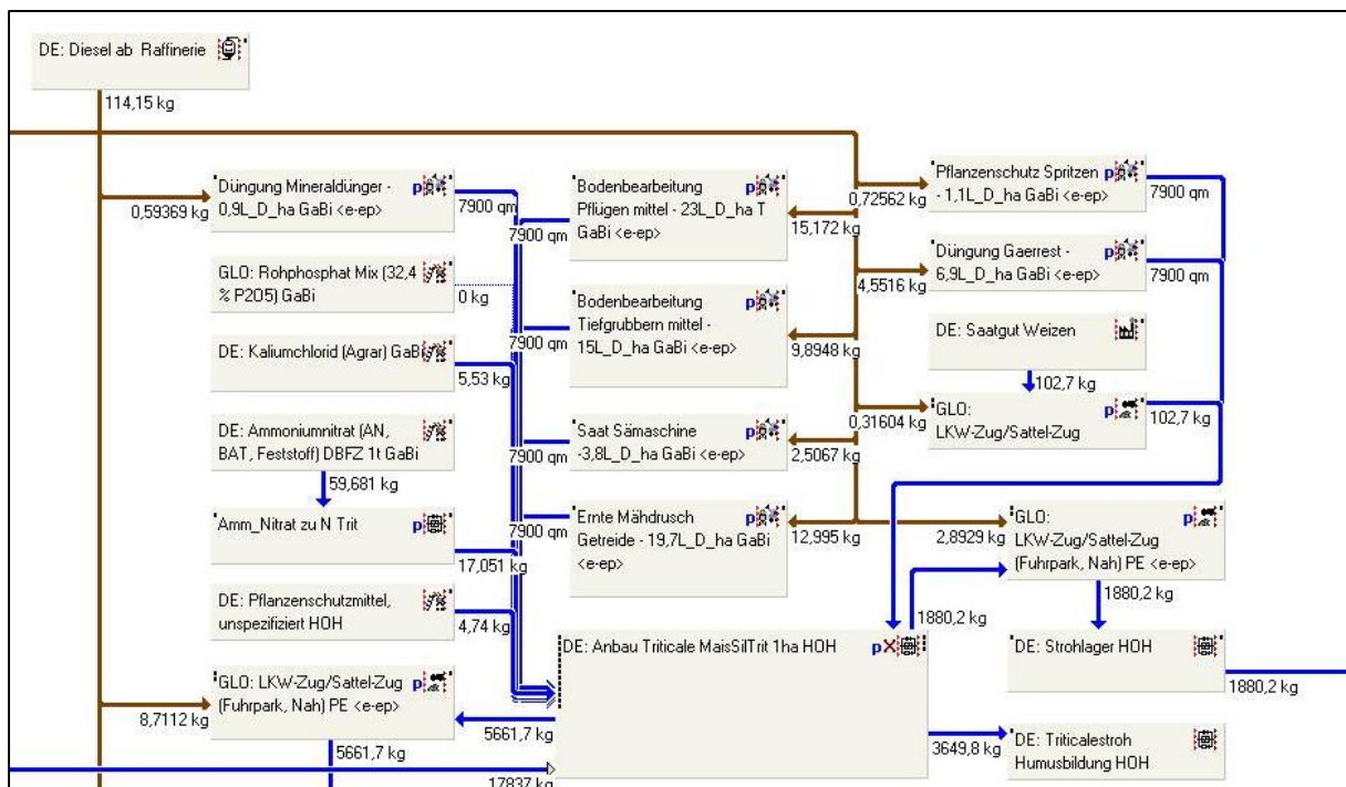
Abb. 12-2: Stoff- und Materialströme Triticaleanbau und Strohernte
