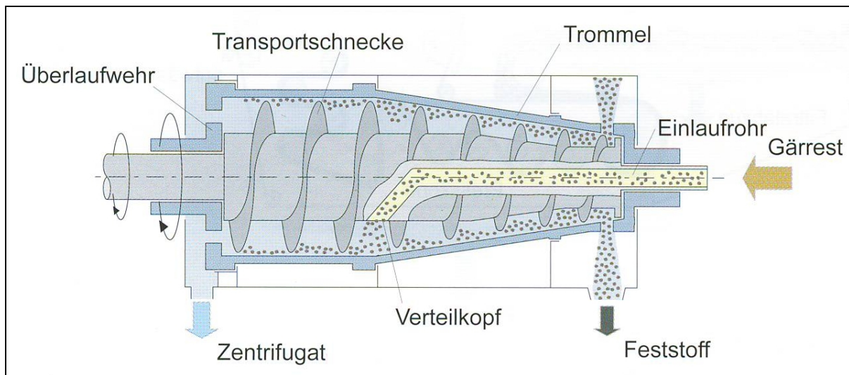
Abb. 10-6: Schematische Darstellung einer Dekanterzentrifuge [20]
